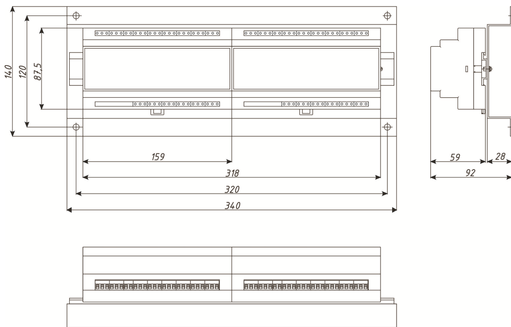
Периферийный блок
